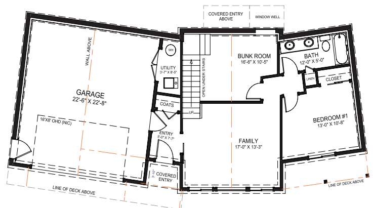
OPTIONAL BASEMENT
