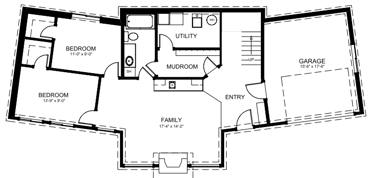
OPTIONAL BASEMENT
